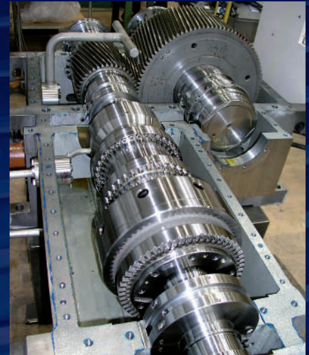
Montage eines Spezialgetriebes Typ G-36s, einschließlich einer HS-26 Synchron-Schaltkupplung, speziell konstruiert für den Antrieb von Gasexpandern.
